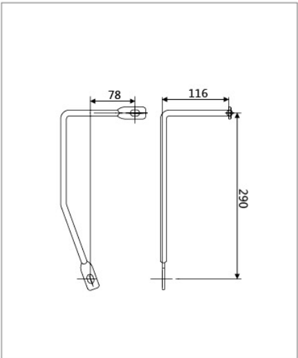
F 单元 C 相母线
