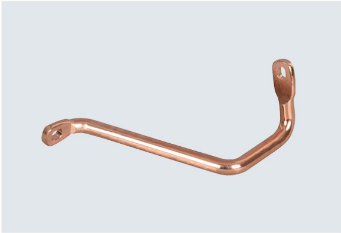
10kV SF6 充气柜 V 单元 C 相母线
