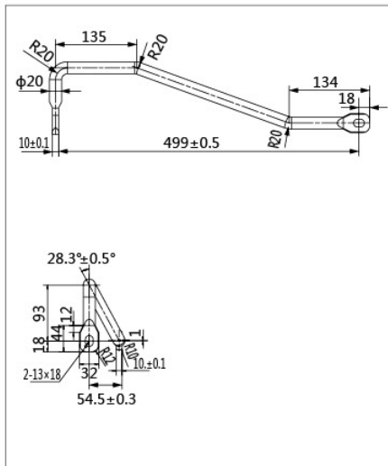
C 单元 B 相母线
