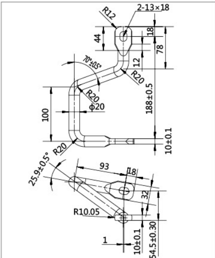
V 单元 B 相母线
