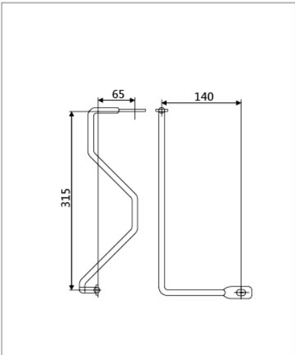
F 单元 B 相母线
