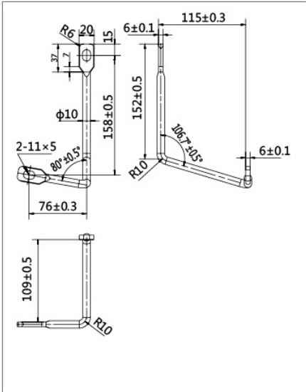
F 单元 A 相母线
