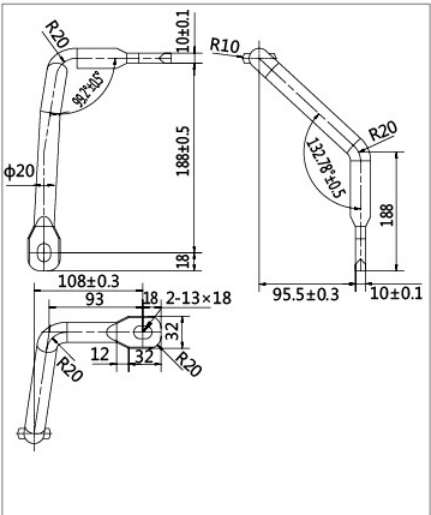
V 单元 C 相母线
