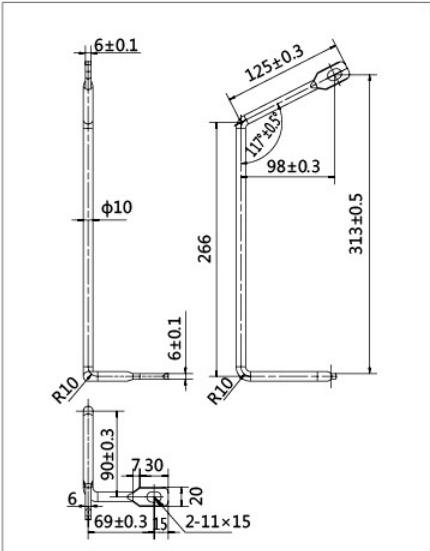
F 单元 B 相母线
